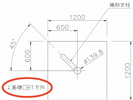
基礎CE2 (平面)
