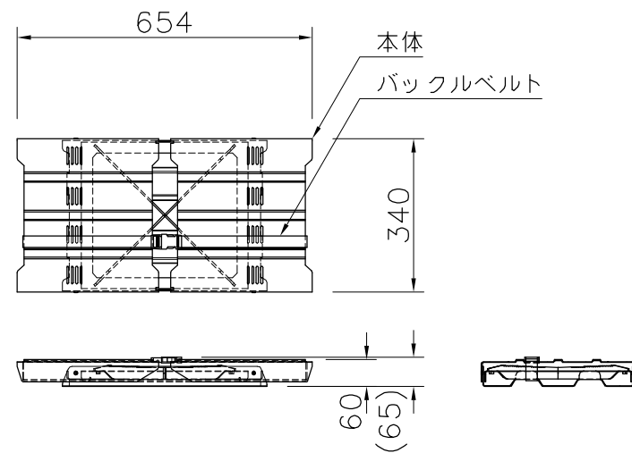
かまど収納状態 外観図 S=1/15
