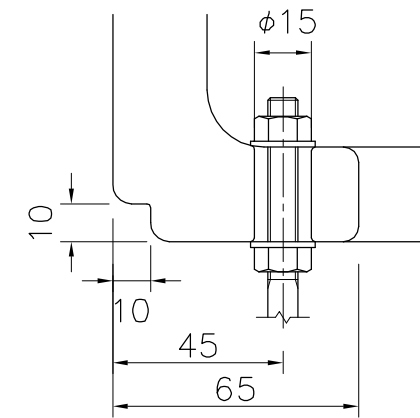
C-C'断面図 S=1/2
