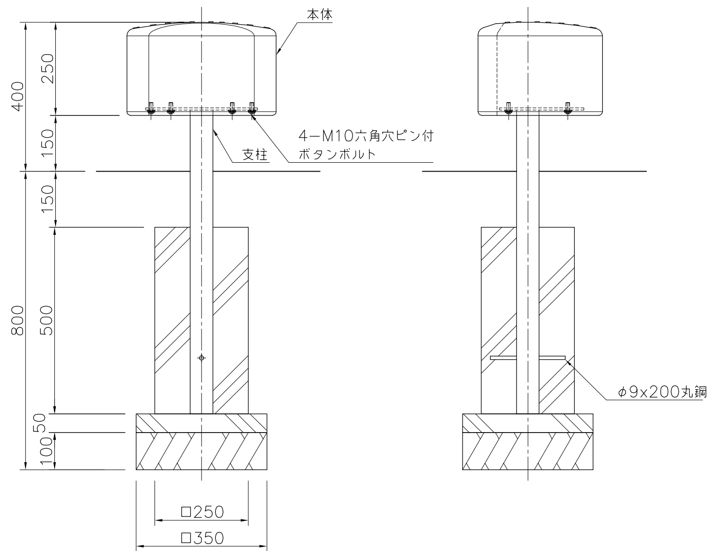
外観図 S=1/10
