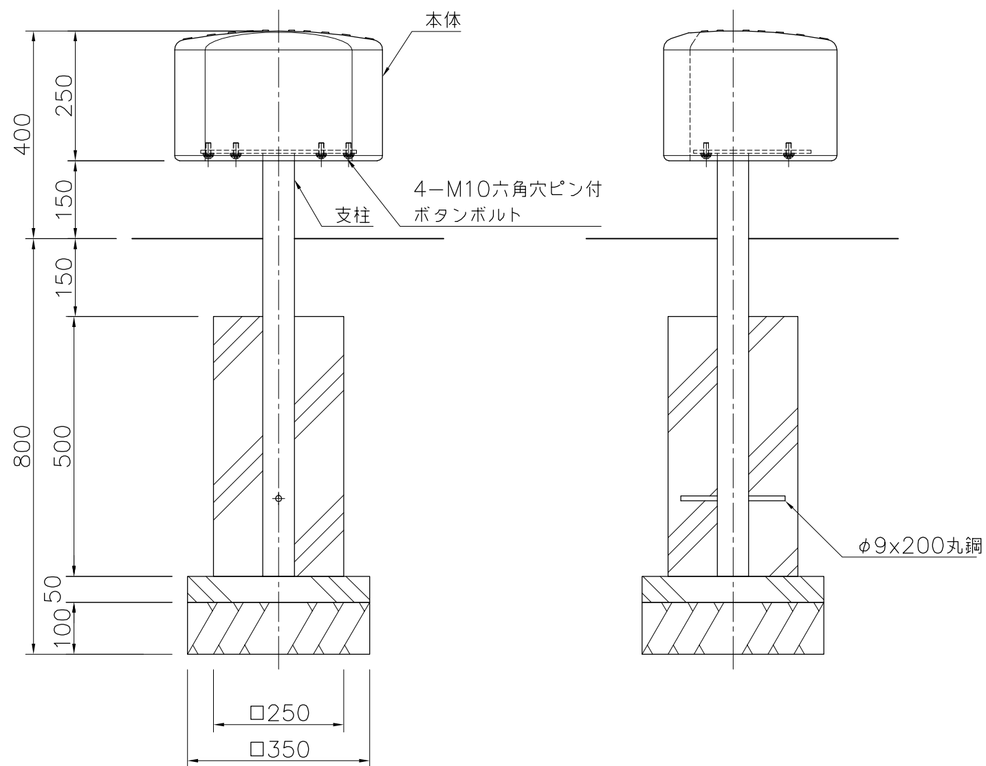
外観図 S=1/10
