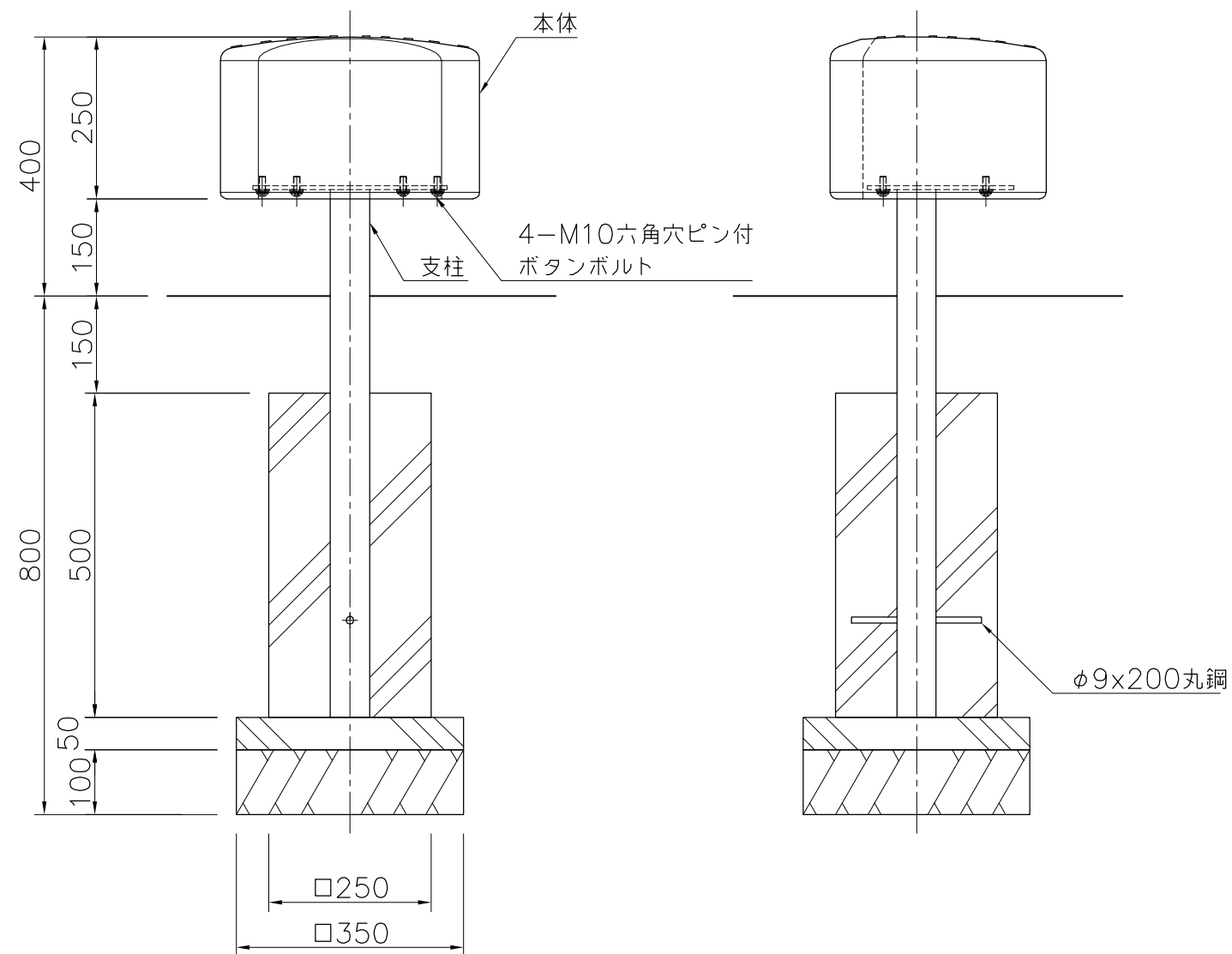
外観図 S=1/10
