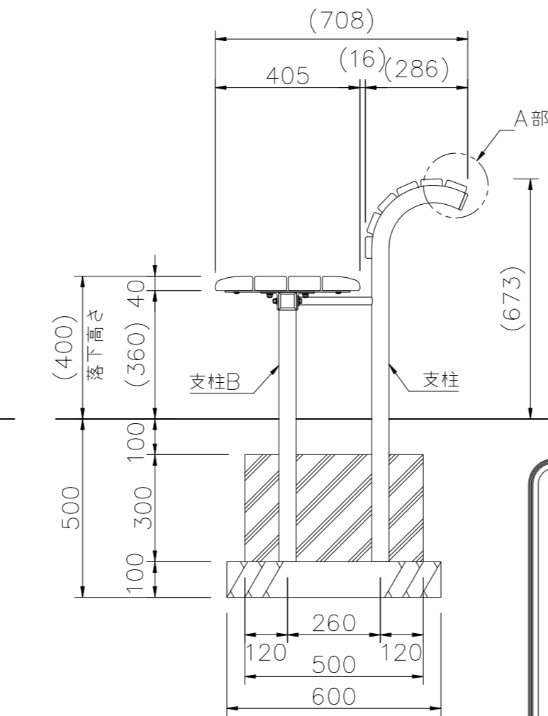
外観図S=1/15
