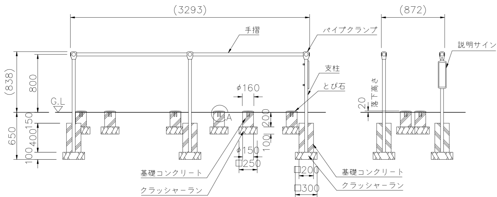
外観図 S=1/30
