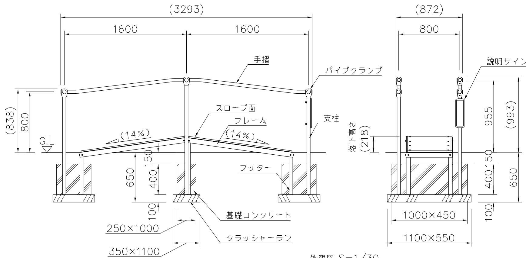
外観図 S=1/30
