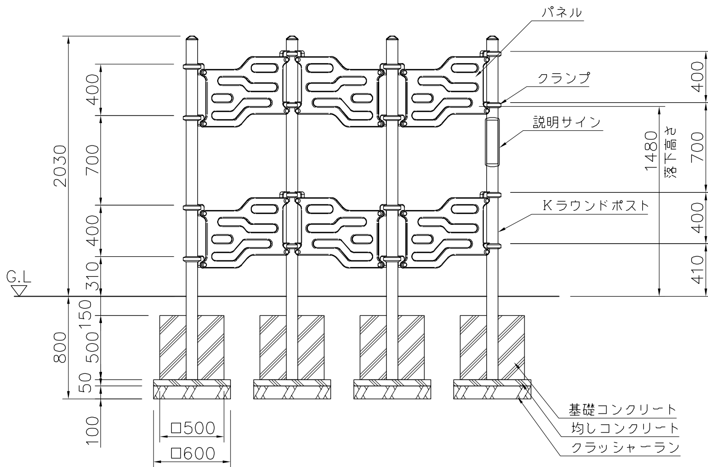
外観図 S=1/30
