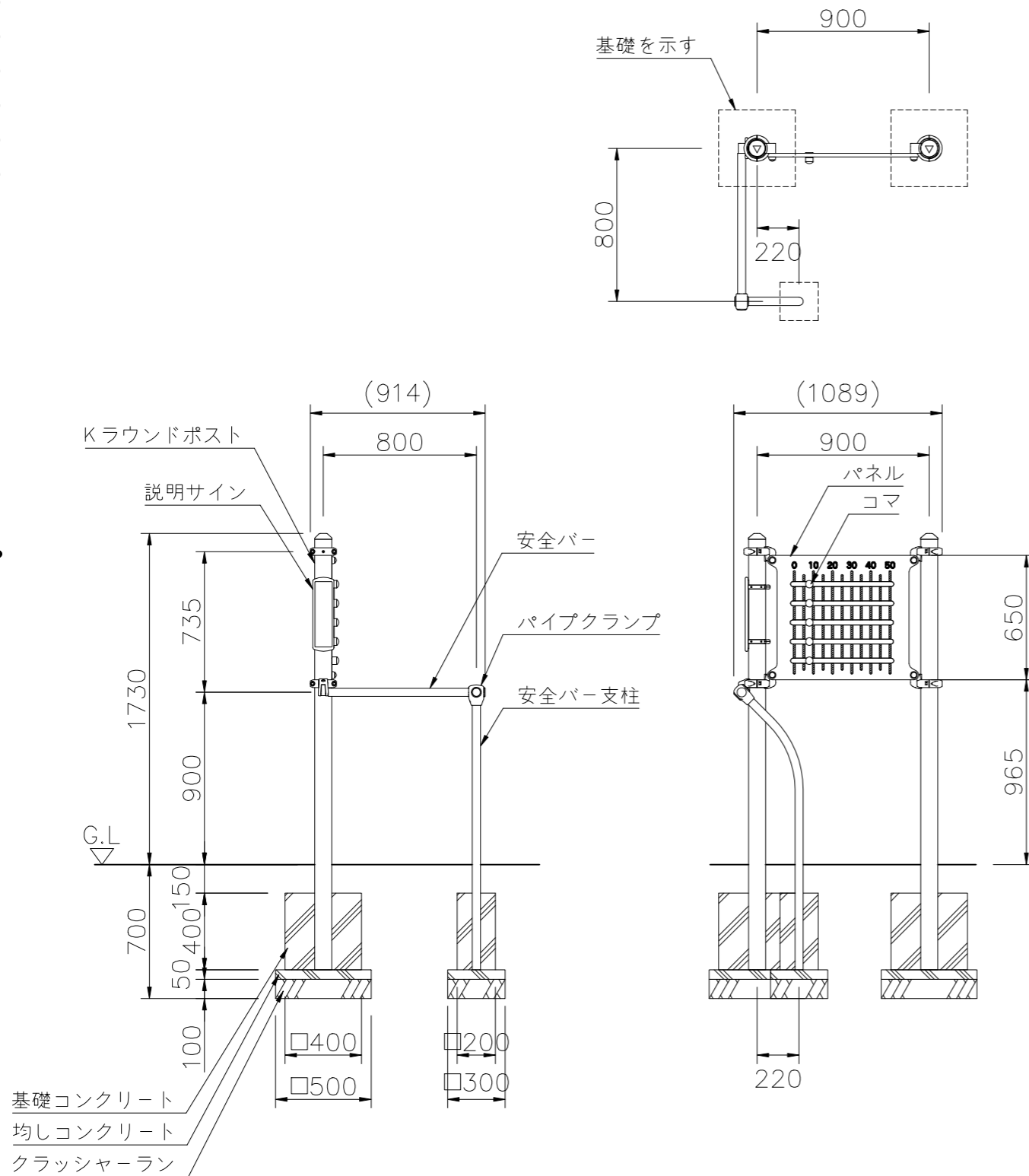
外観図 S=1/30
