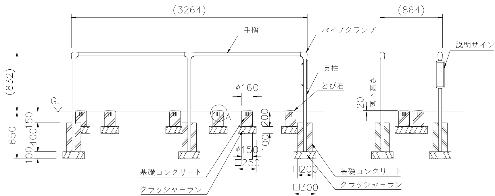
外観図 S=1/30
