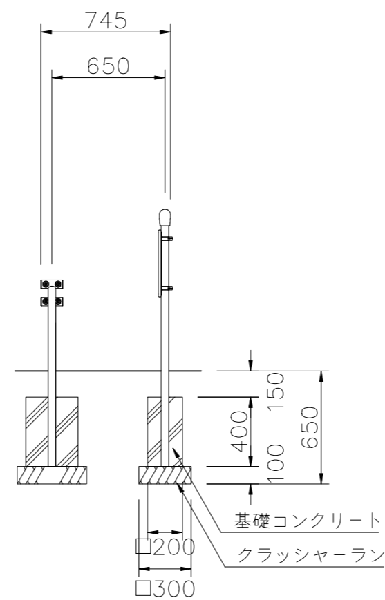
外観図 S=1/30
