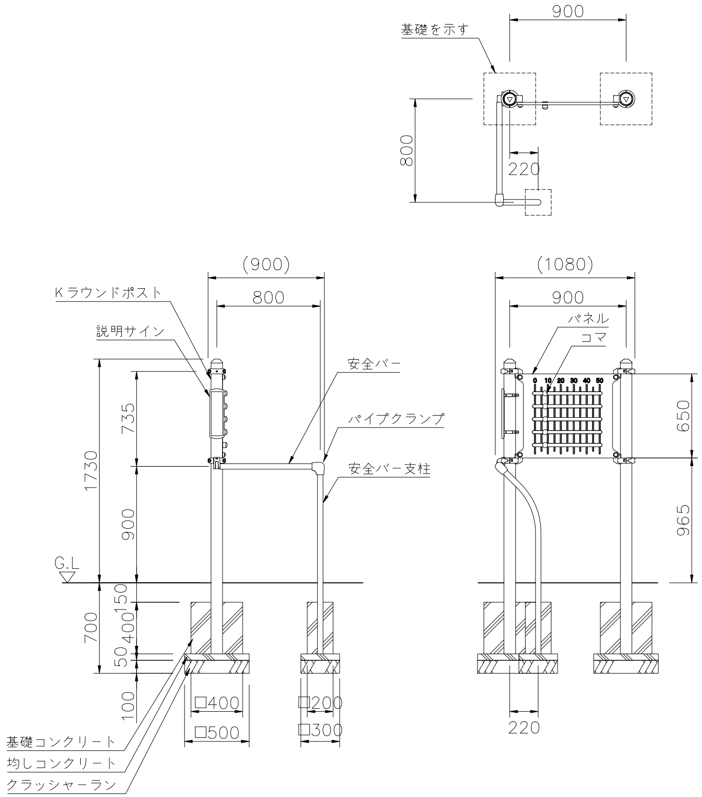
外観図 S=1/30
