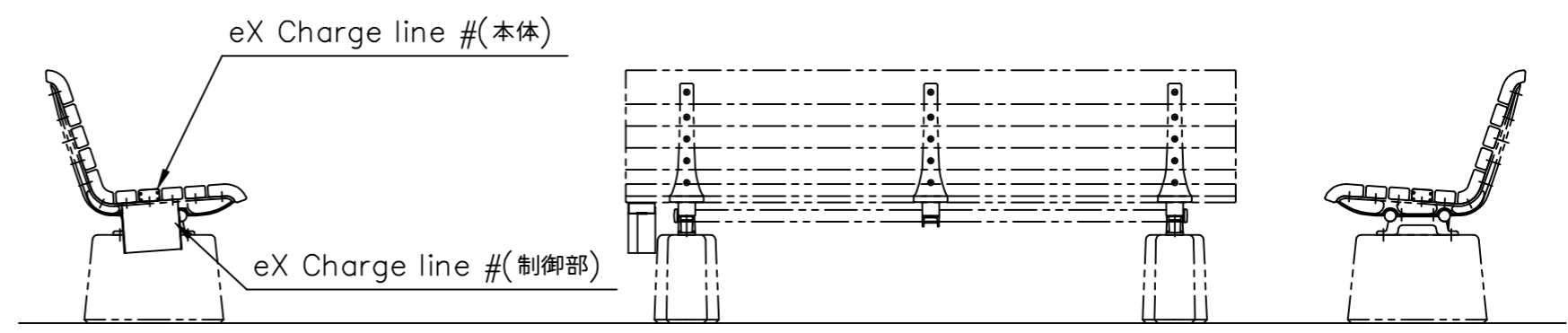
ベンチ取付参考図 S=1/20
