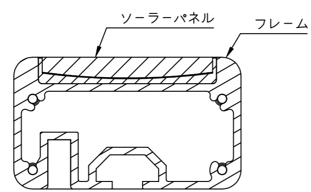
A-A 断面図 S=1/1
