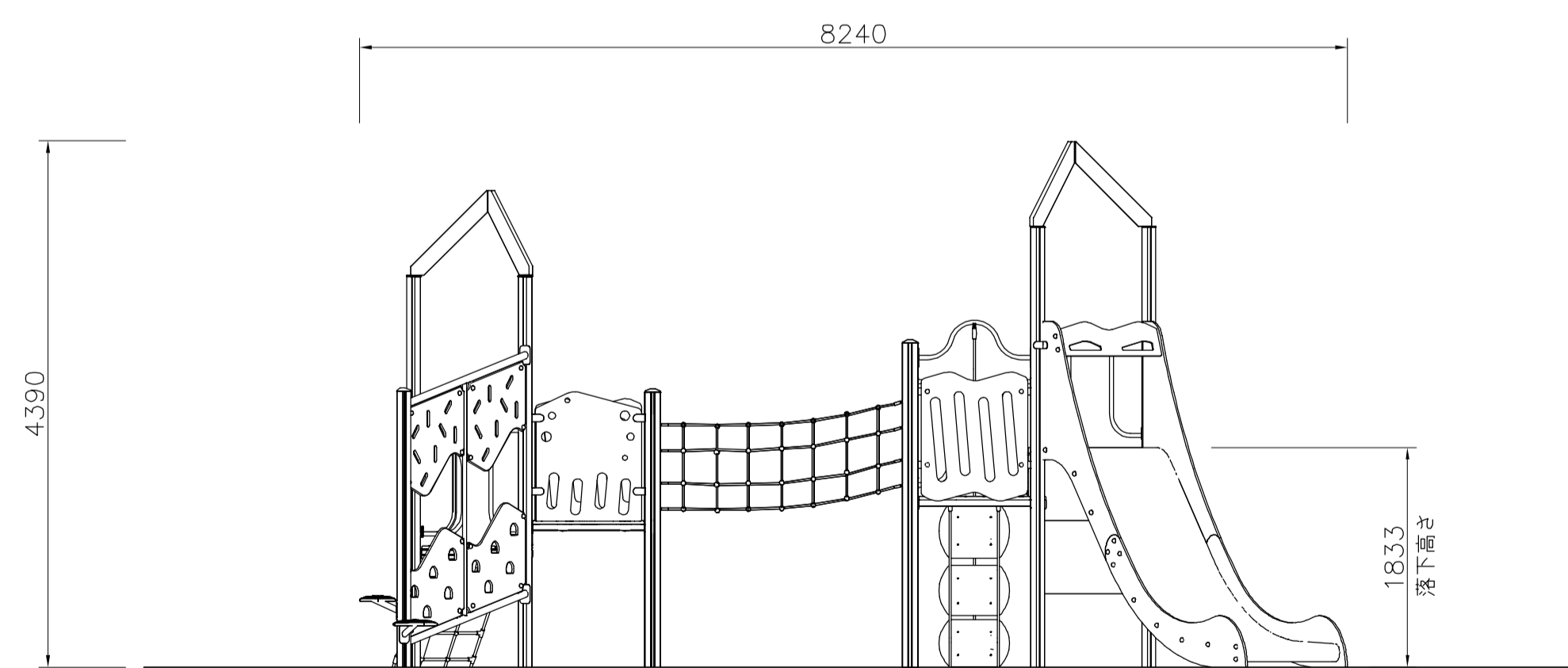
外観図 S=1/50
