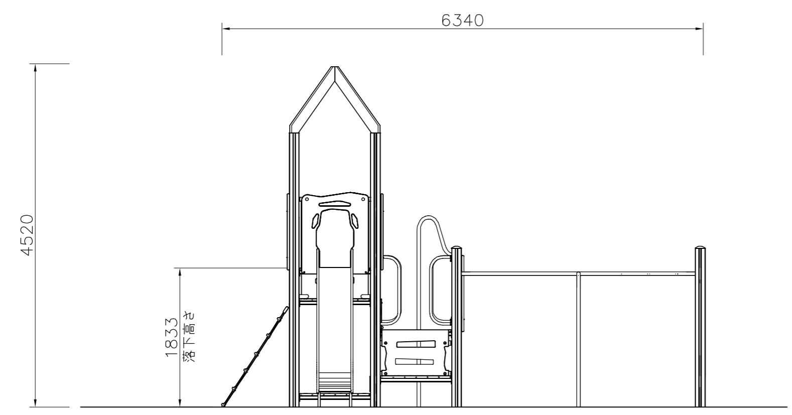
外観図 S=1/50
