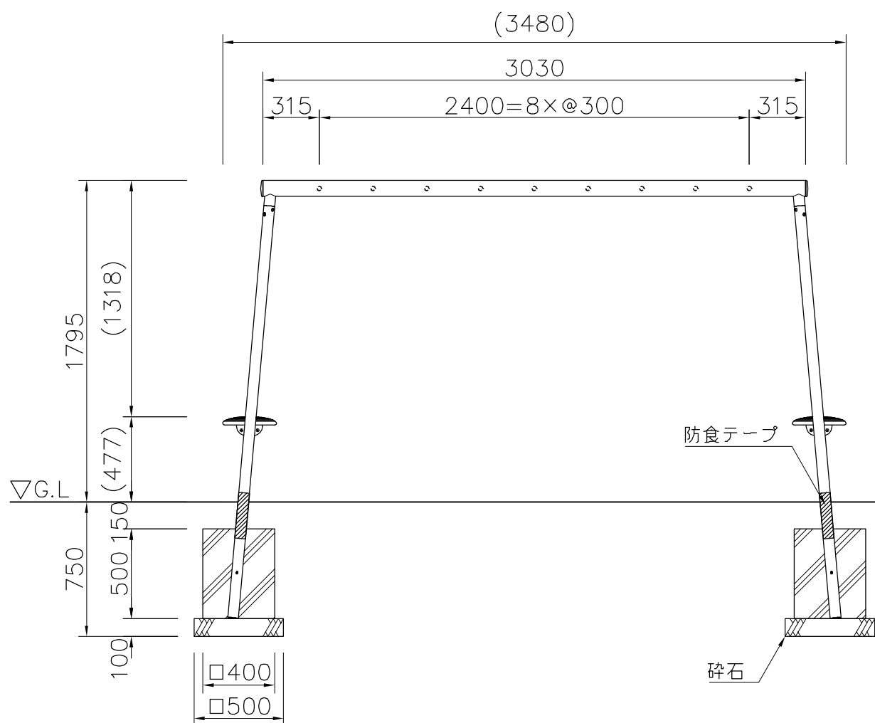
外観図 S=1/30
