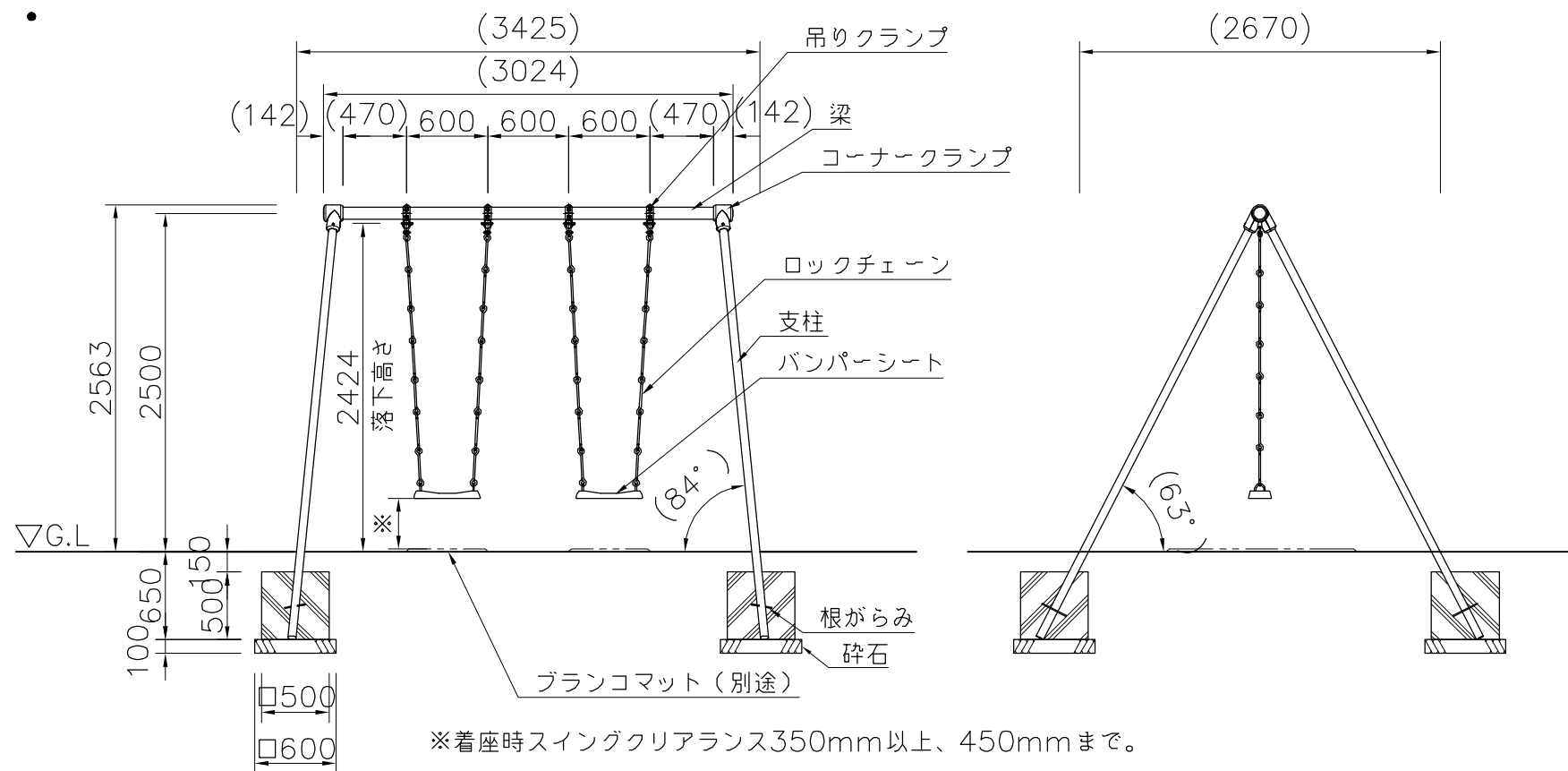
外観図 S=1/50
