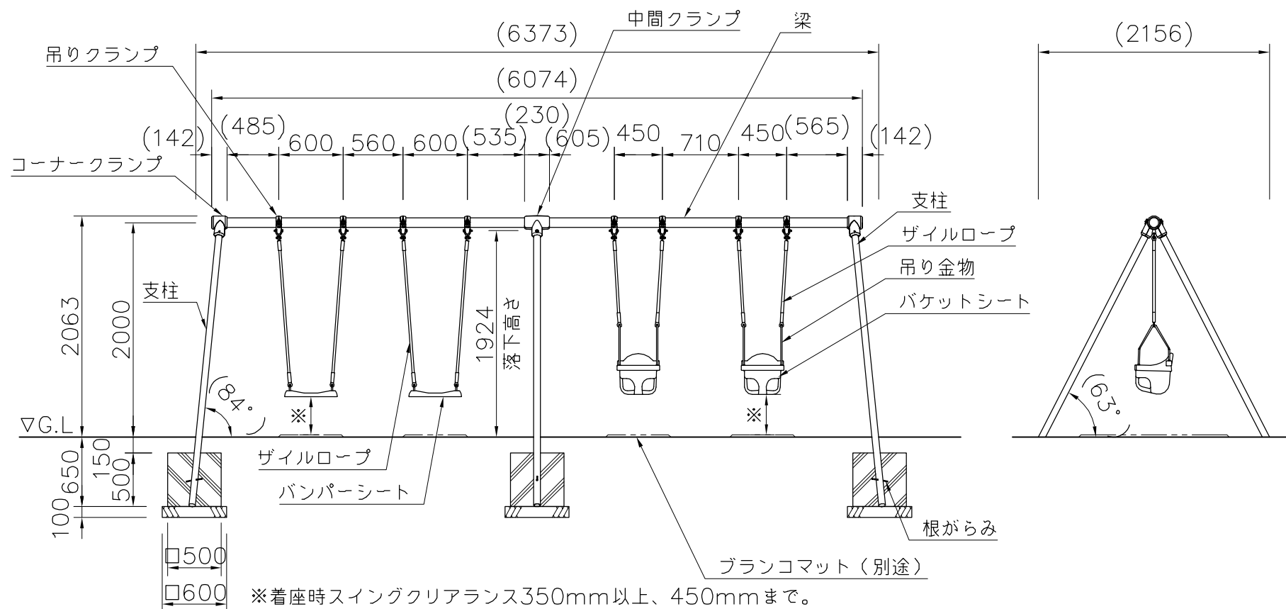
外観図 S=1/50
