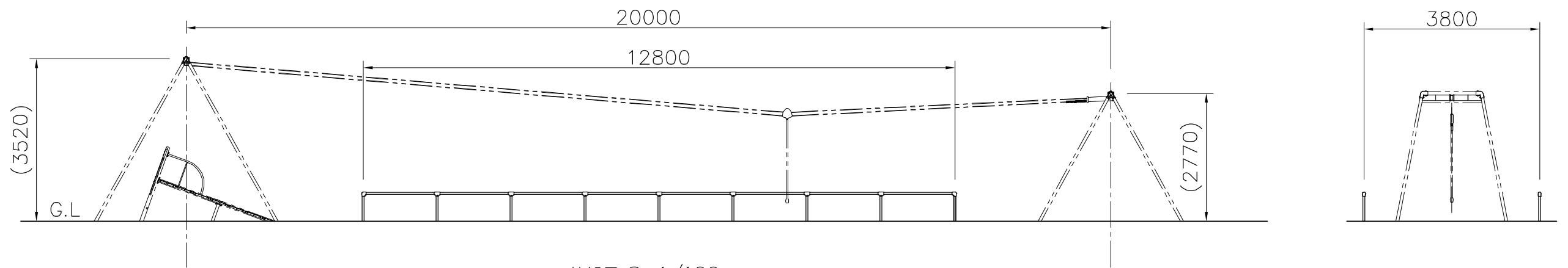
外観図 S=1/100
