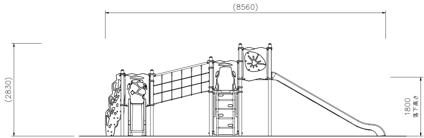
外観図 S=1/50
