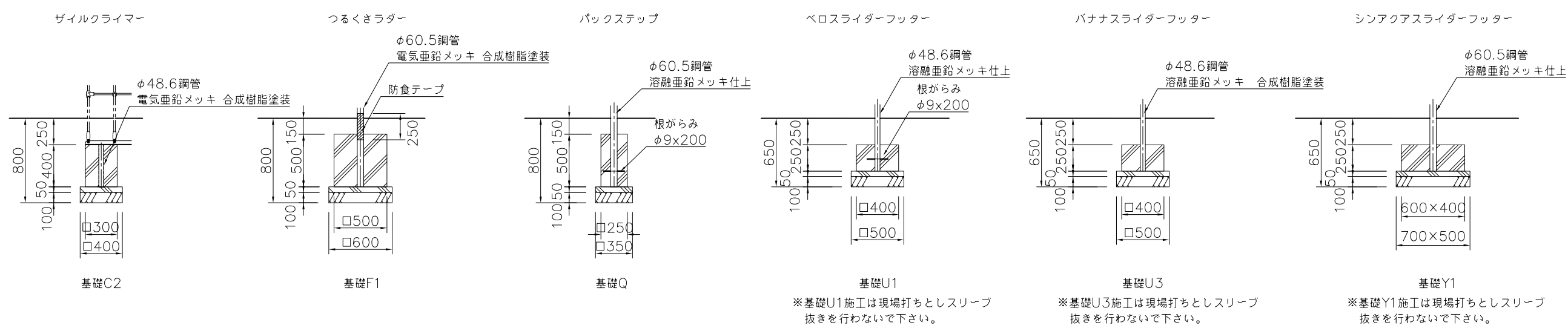
基礎詳細図 S=1/30
