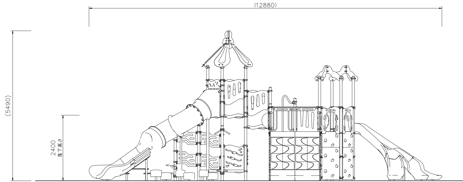
A 矢視
