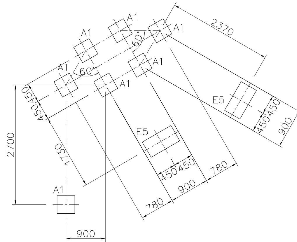
基礎伏図 S=1/50
