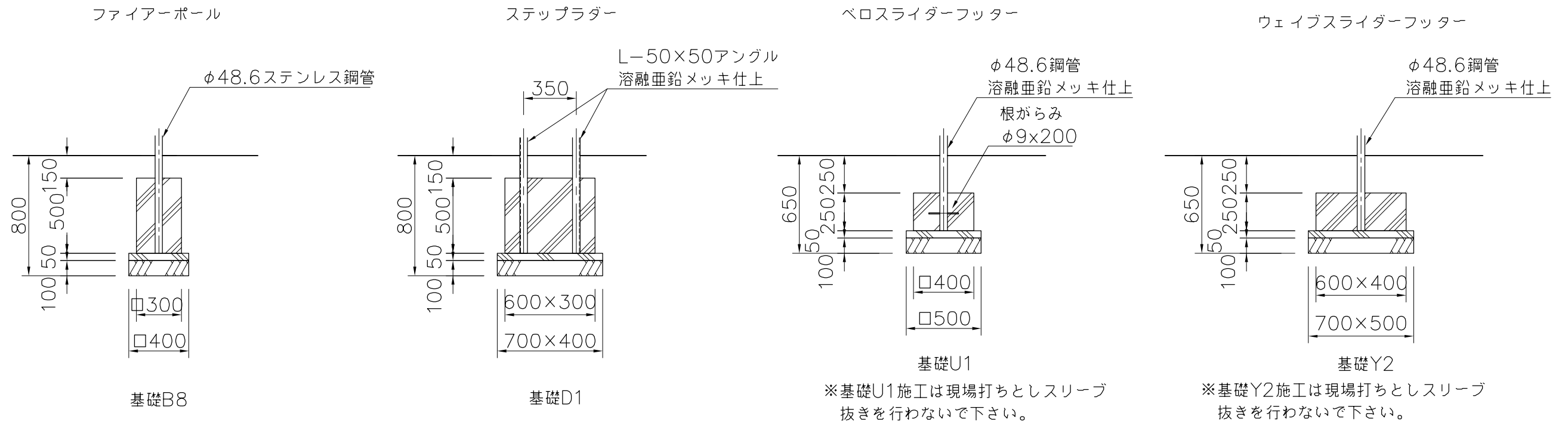
基礎詳細図 S=1/30
