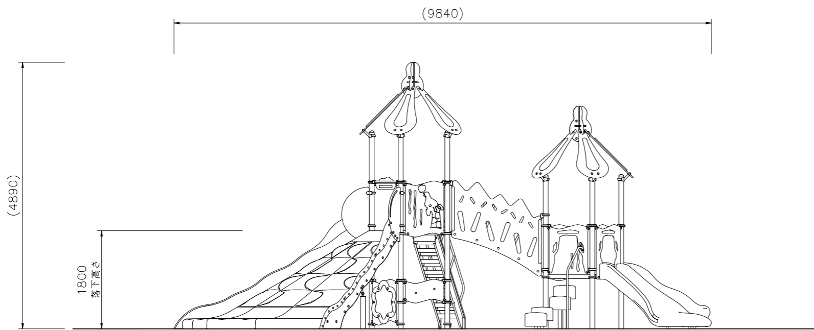
外観図 S=1/50
