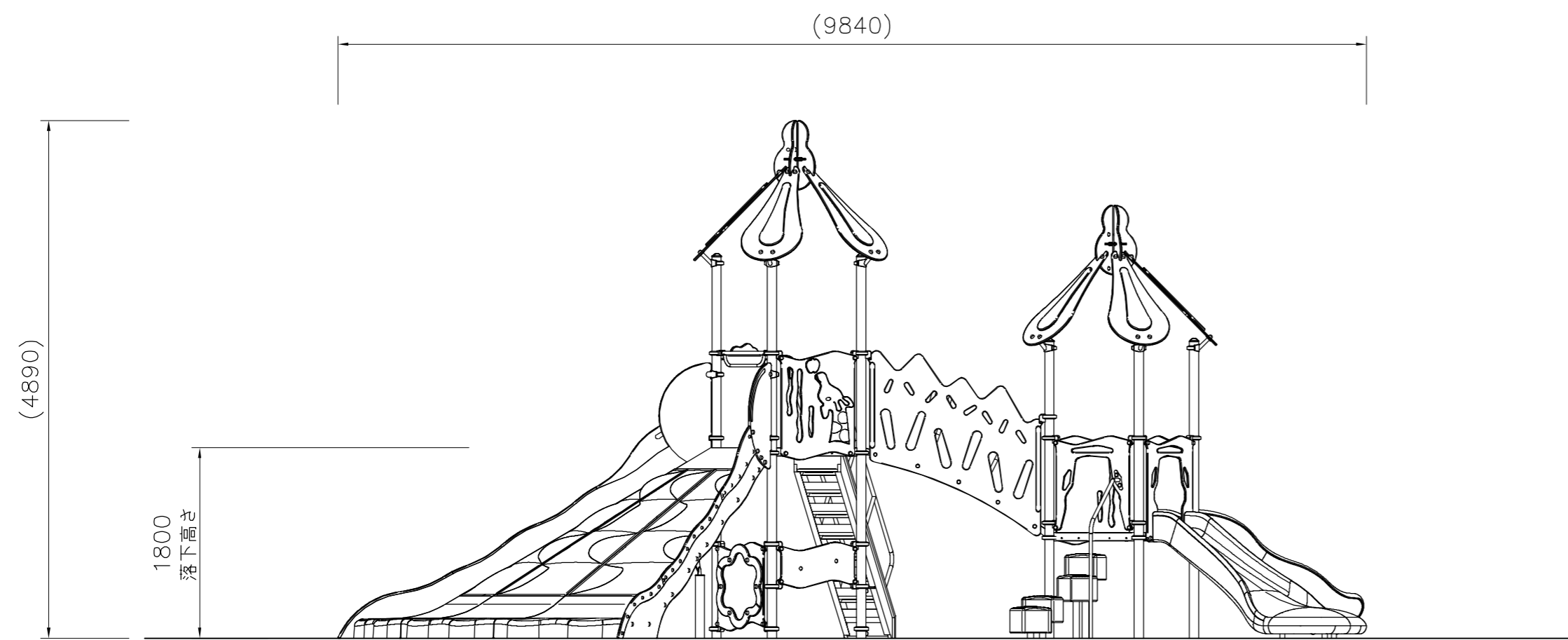
外観図 S=1/50
