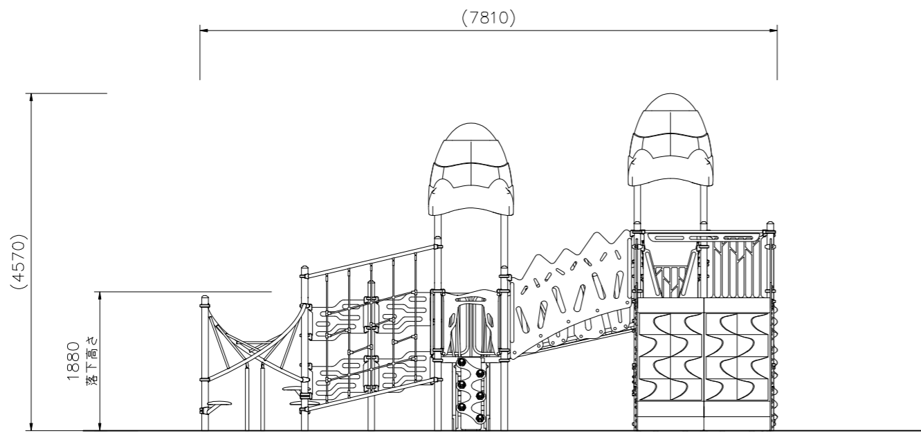
A 矢視
