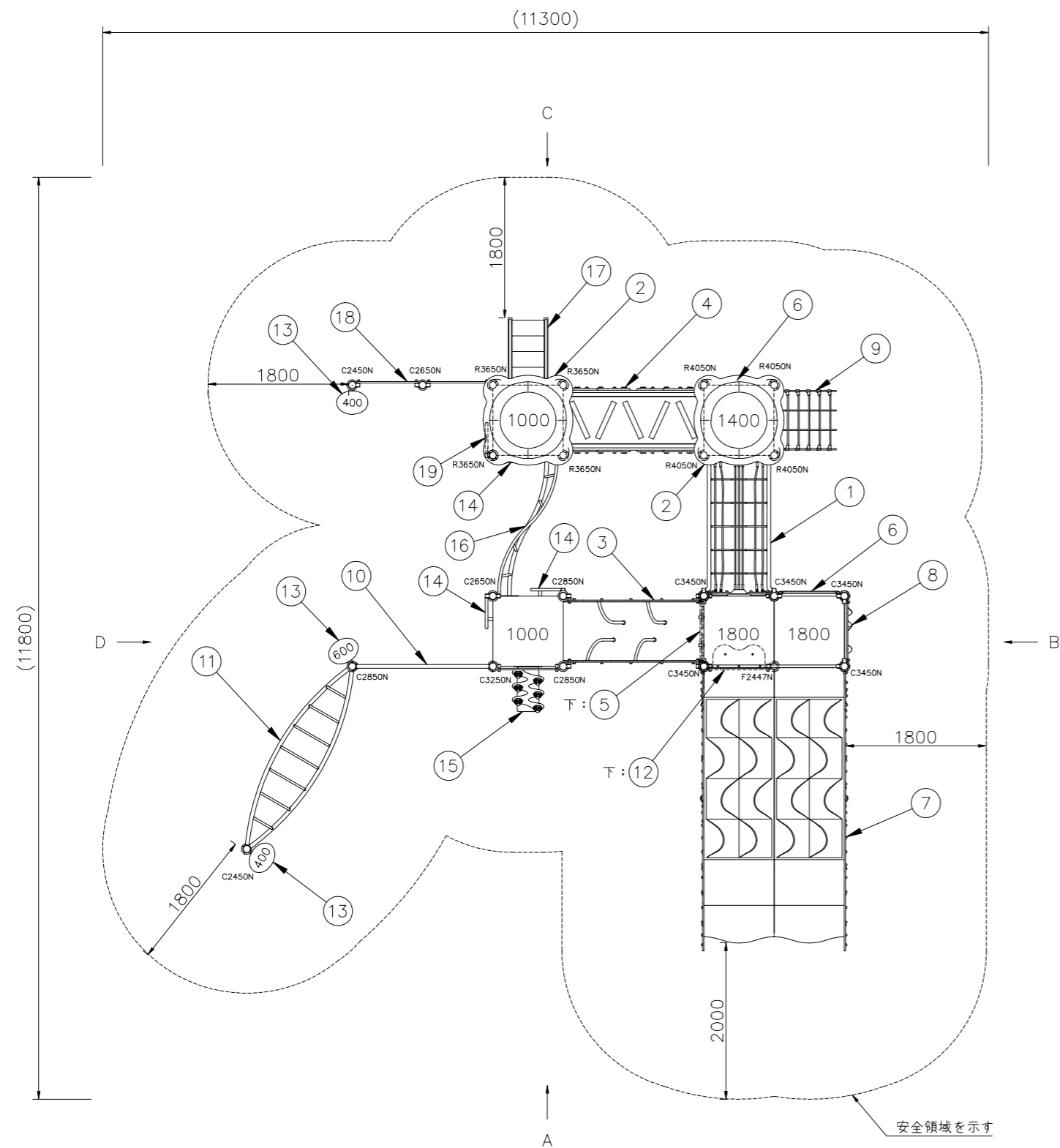
平面図 S=1/50
