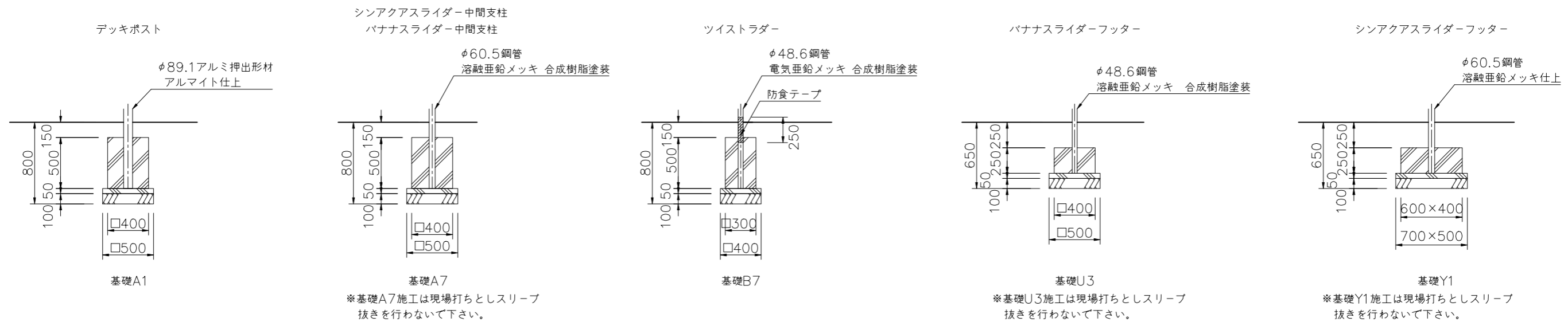
基礎詳細図 S=1/30
