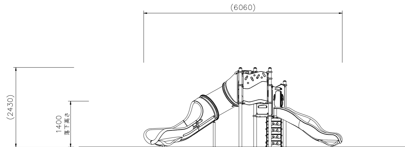
外観図 S=1/50
