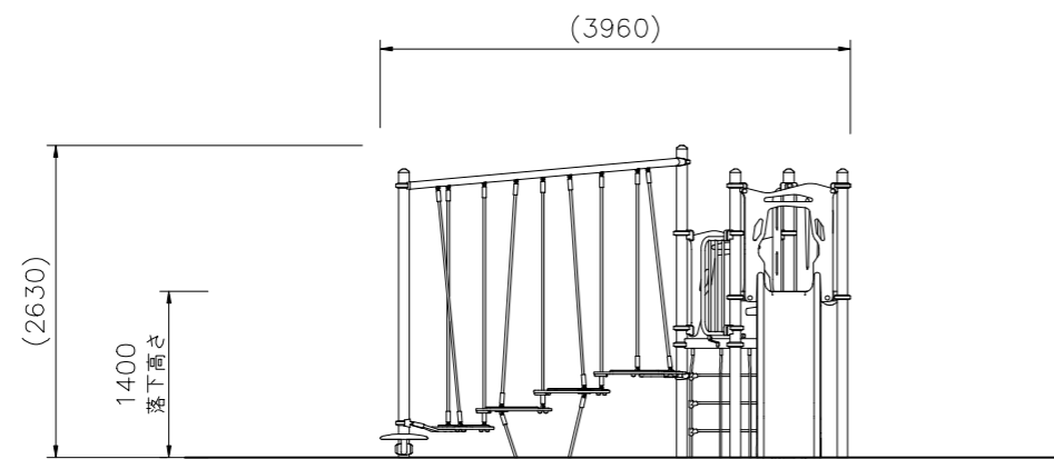
外観図 S=1/50
