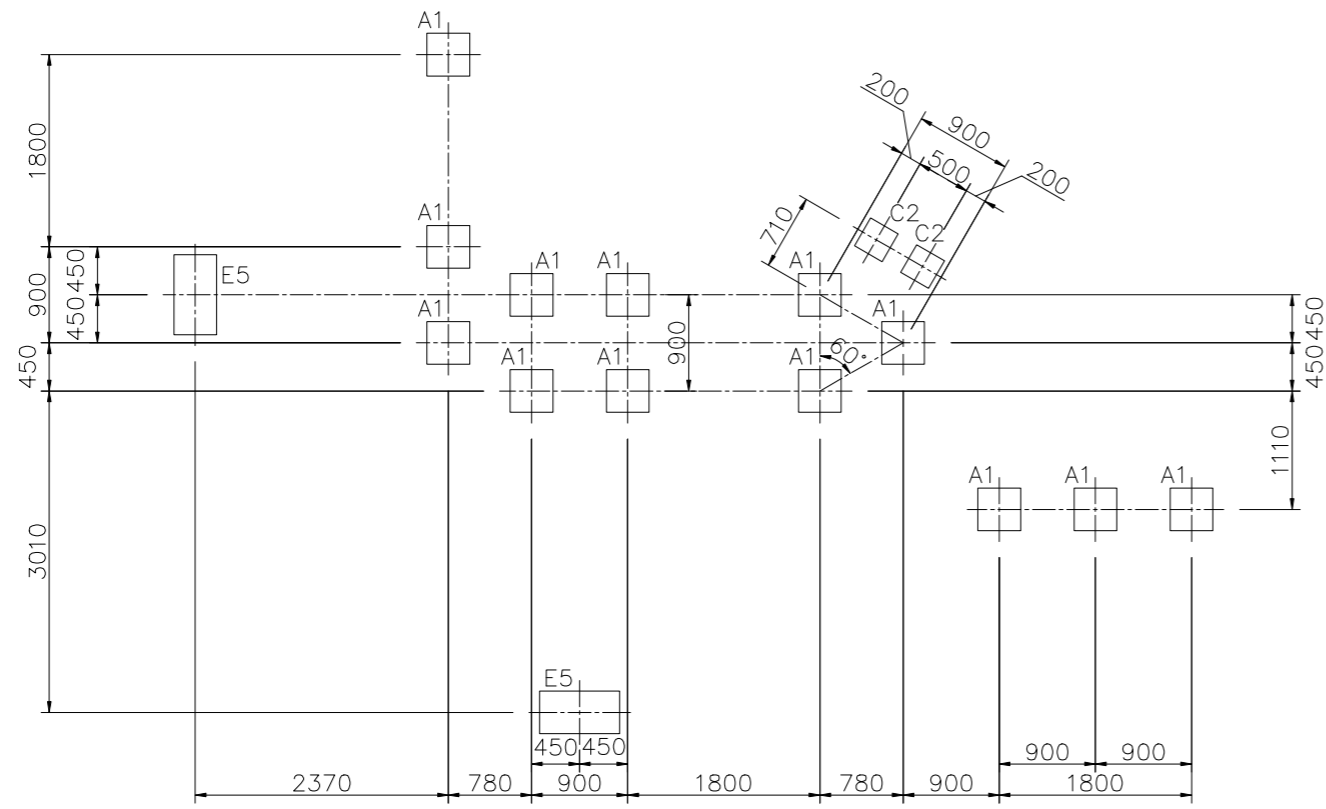
基礎伏図 S=1/50
