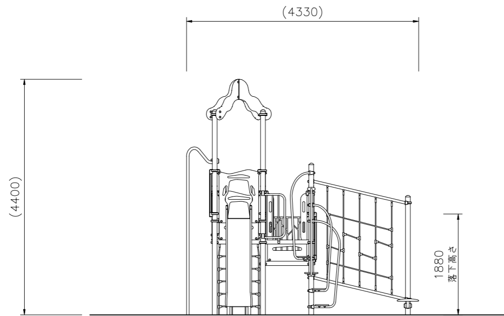
外観図 S=1/50
