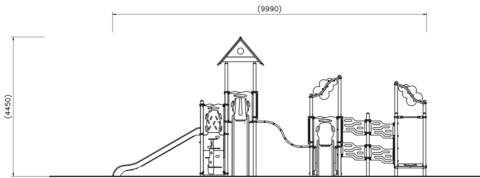
外観図 S=1/50
