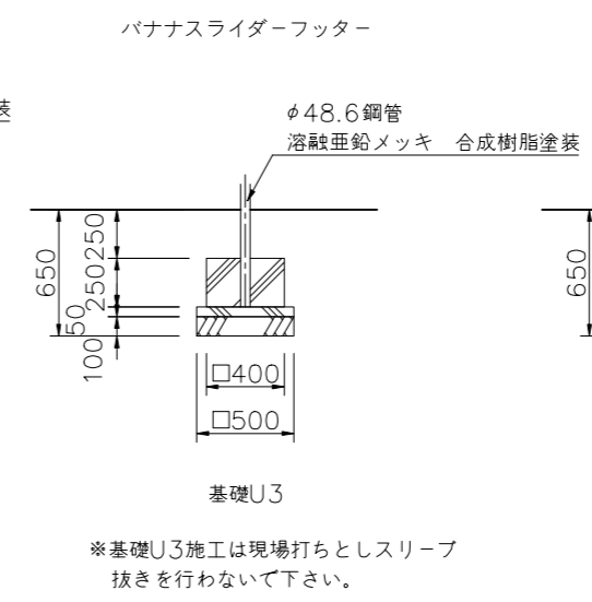
基礎詳細図 S=1/30
