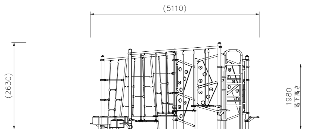
外観図 S=1/50
