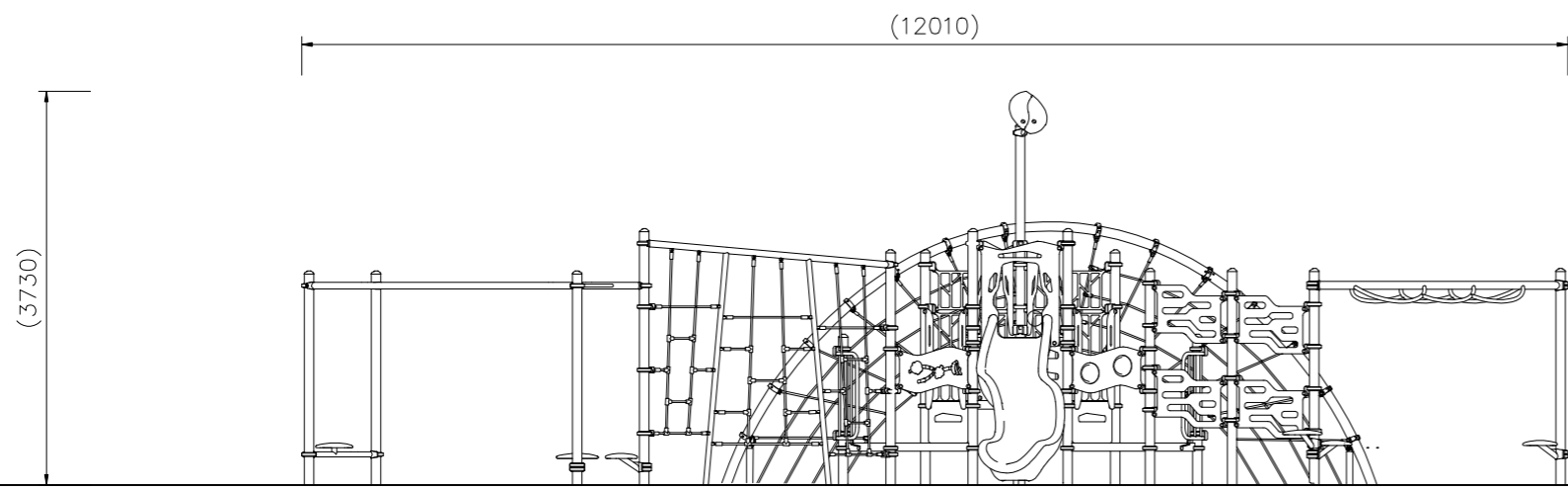
外観図 S=1/50
