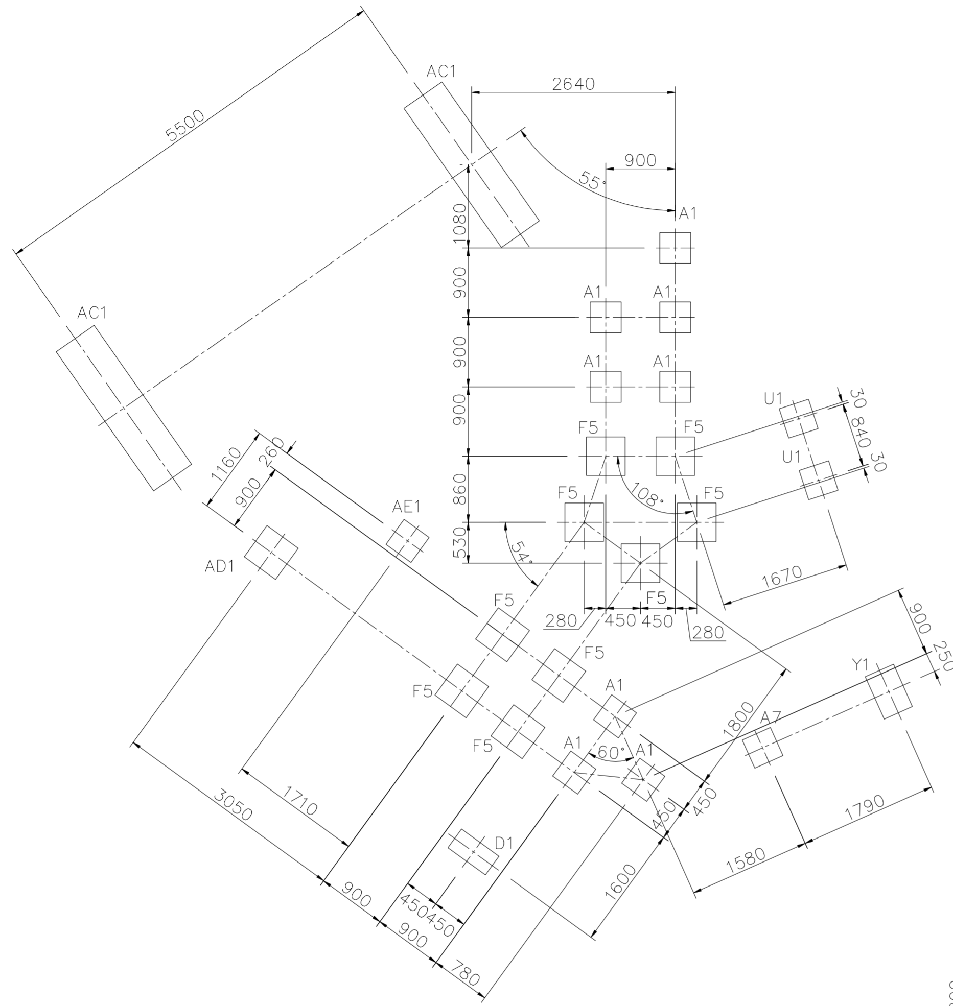
基礎伏図 S=1/50
