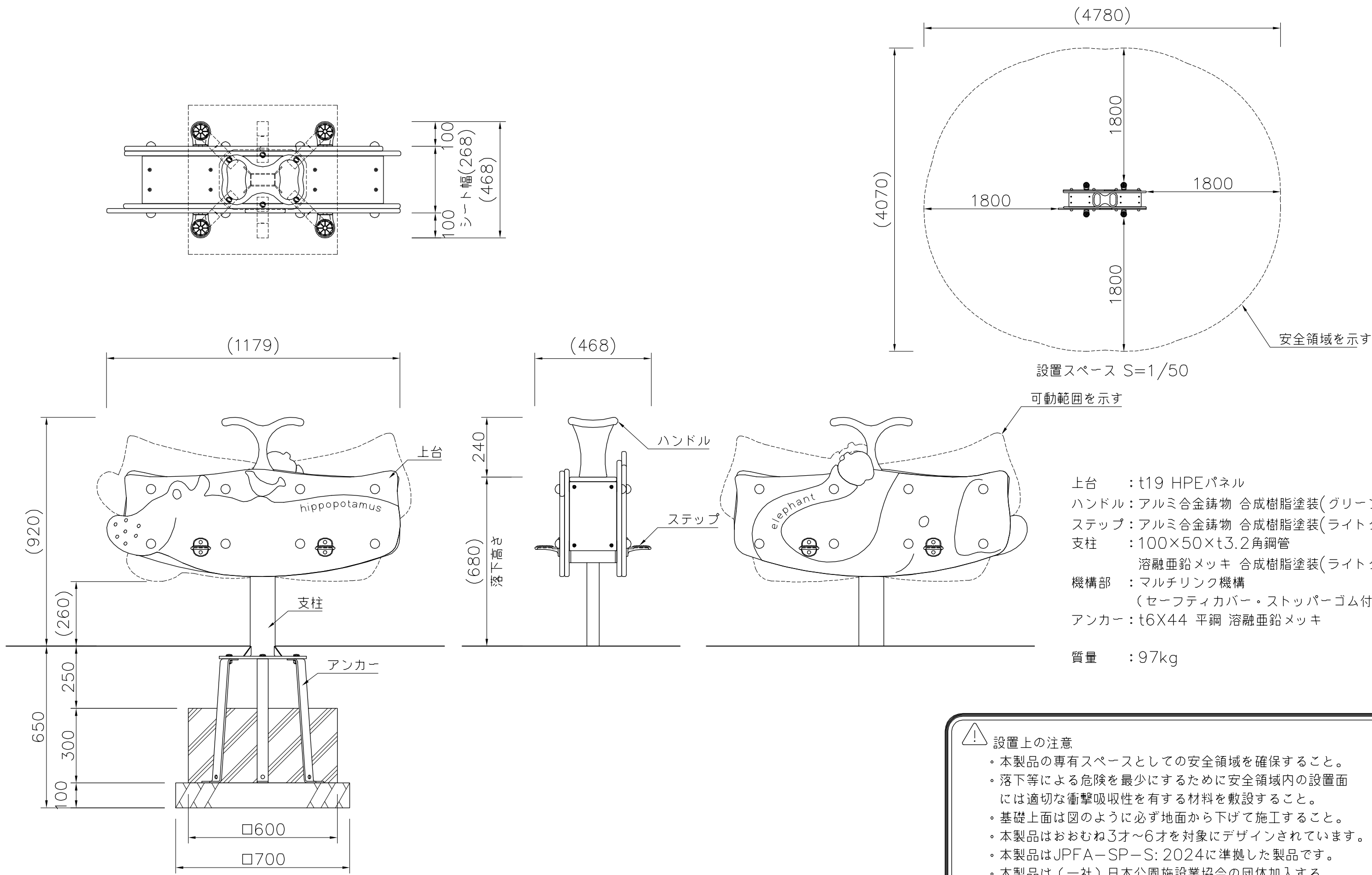
外観図 S=1/15
