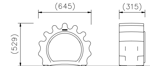
詳細図 S=1/20
