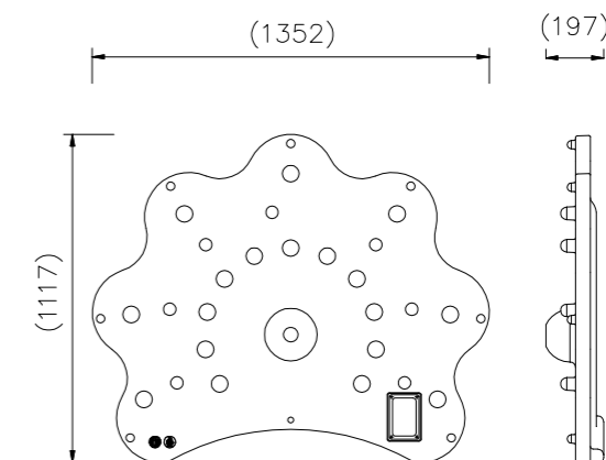
詳細図 S=1/20
