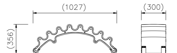
詳細図 S=1/20
