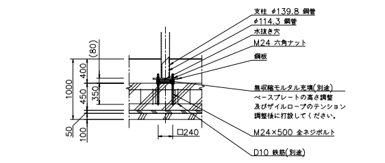
基礎CB1 詳細図い
