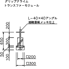
基礎CH1
