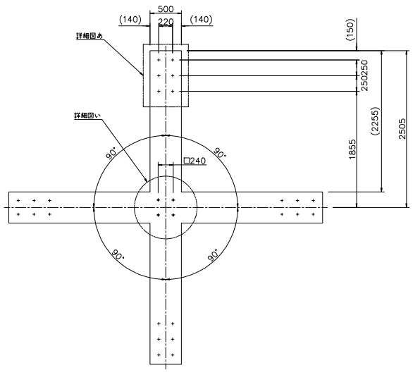
基礎CB1 (平面)
