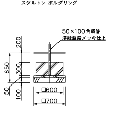
基礎CG1
