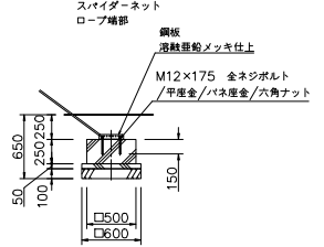
基礎CJ3
