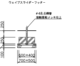
基礎Y2 *基礎Y2施工は現場打ちとしスリーブ抜きを行わないで下さい。
