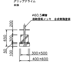
基礎CH2
