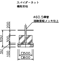
基礎CJ2
