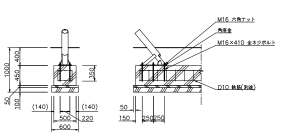
基礎CB1 詳細図め
