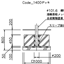
基礎CE1
