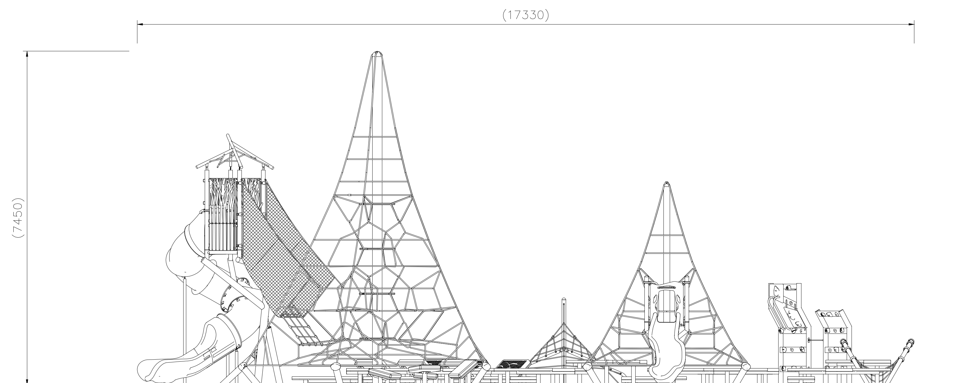
B 矢視
