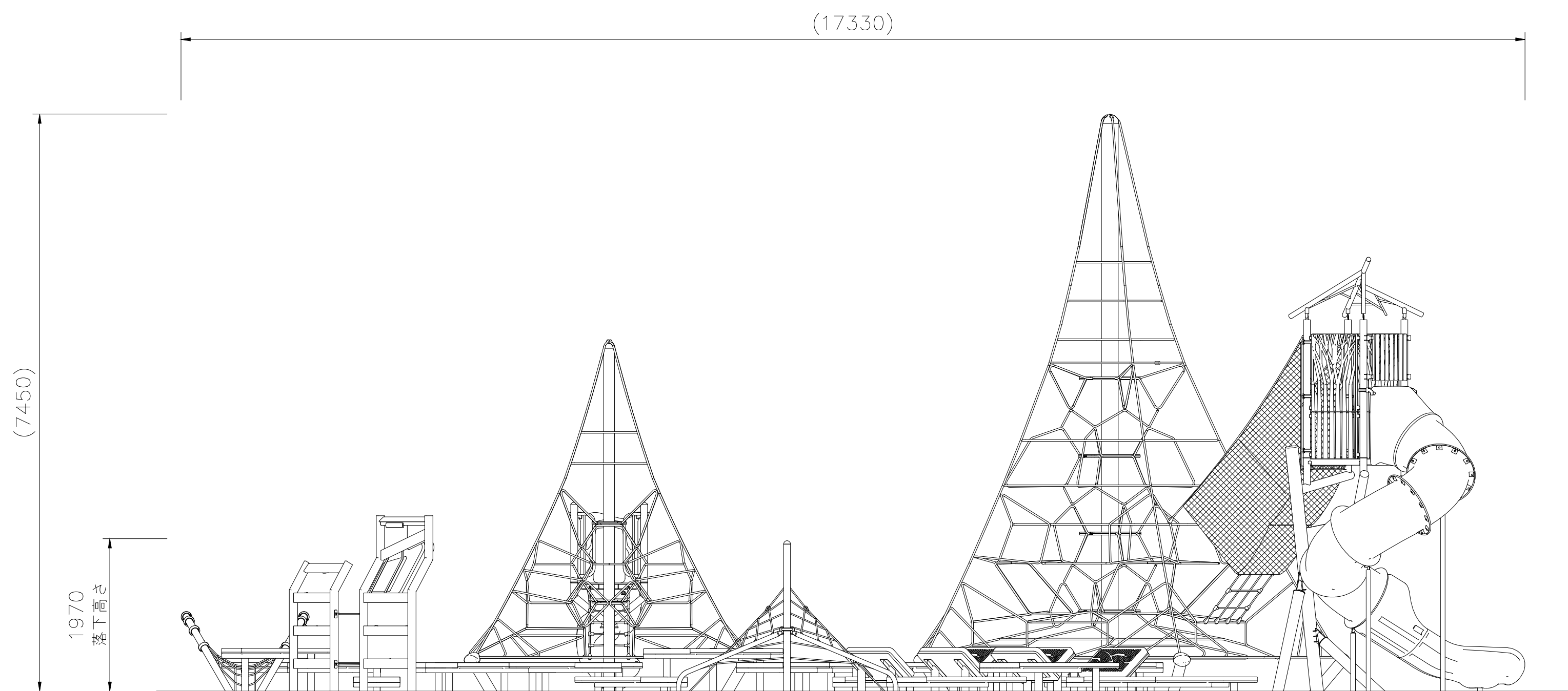
D 矢視
