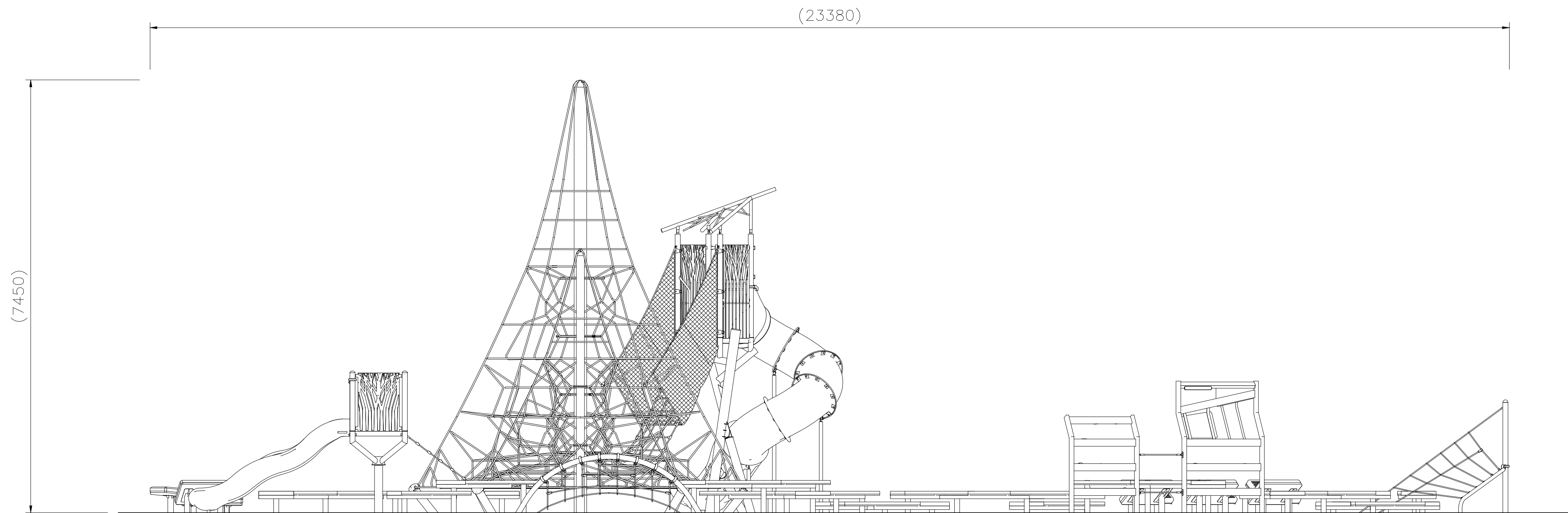
C 矢視
