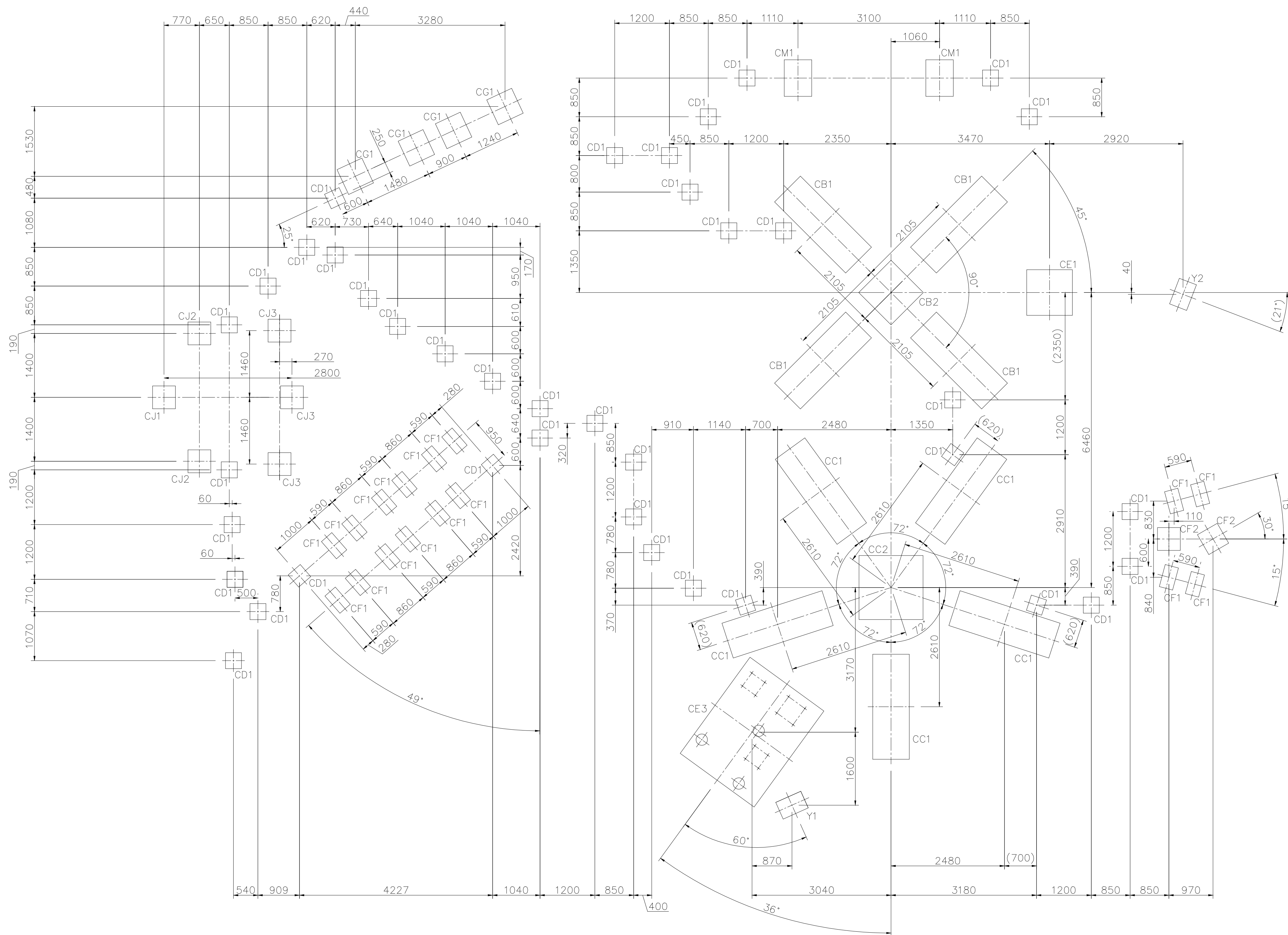
基礎図 S=1/50
