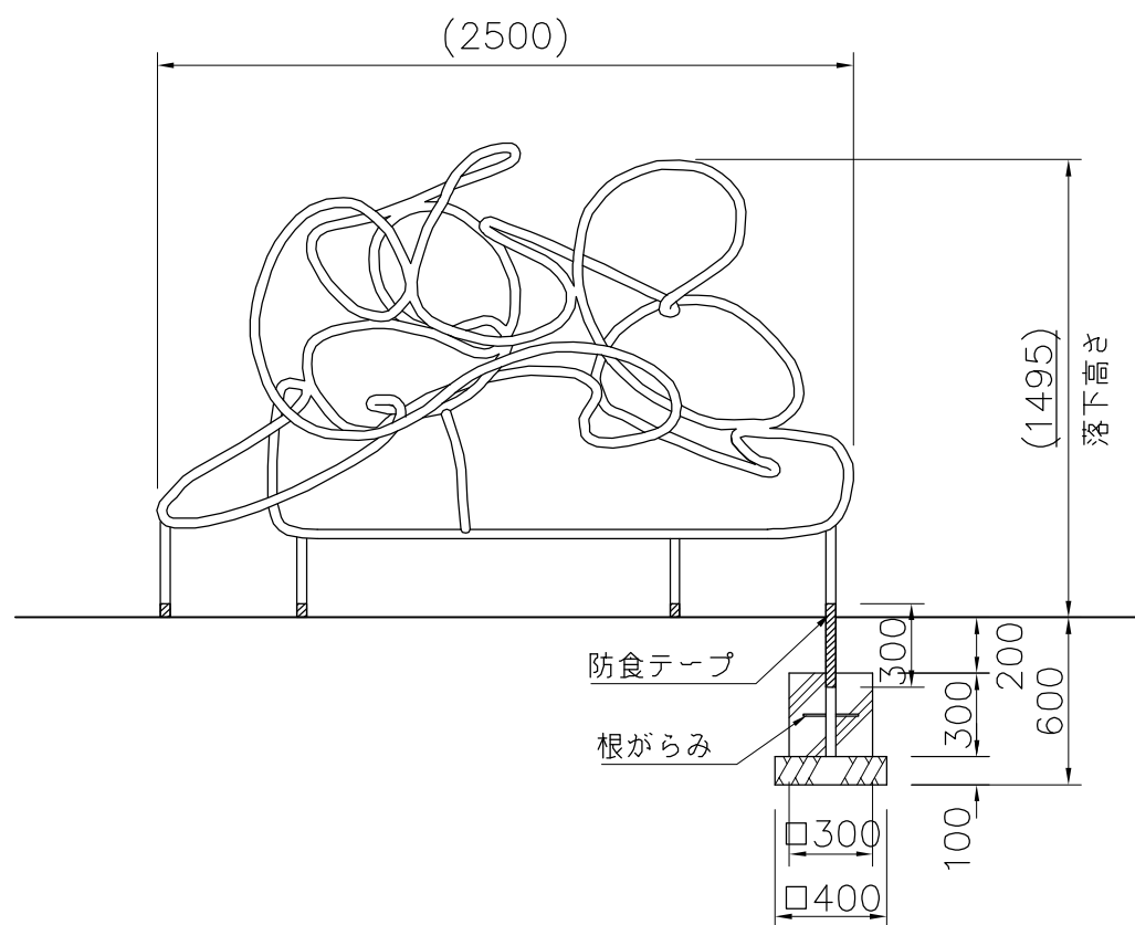
外観図 S=1/30
