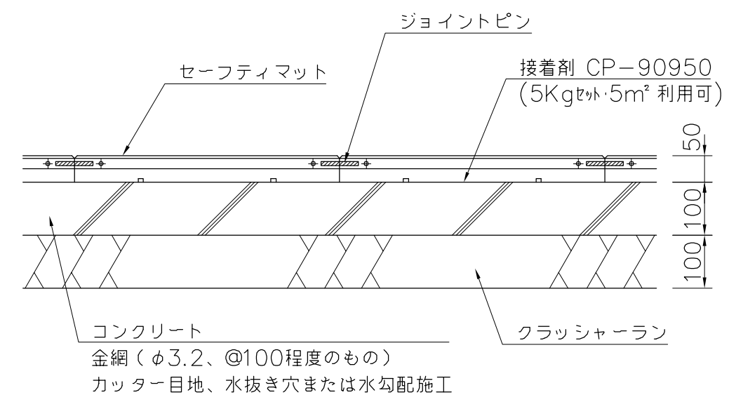
参考施工図 S = 1 / 10
