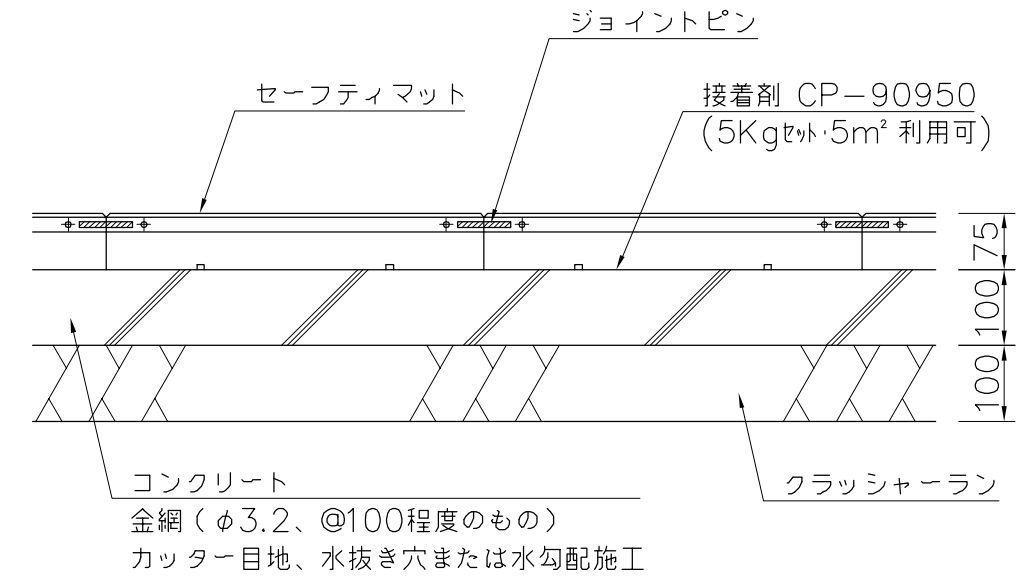
参考施工図 S = 1 / 10
