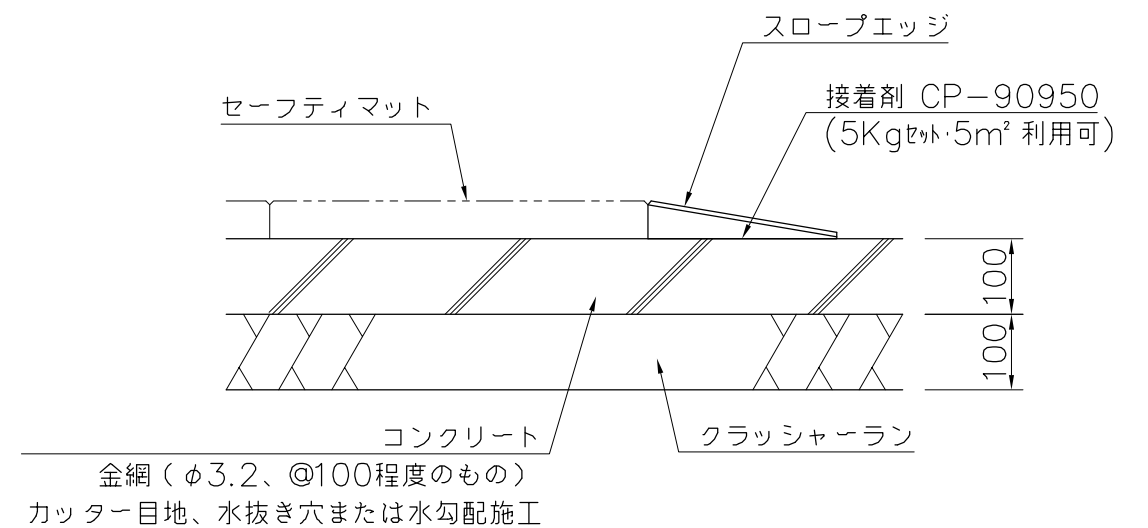
参考施工図 S = 1 / 10
