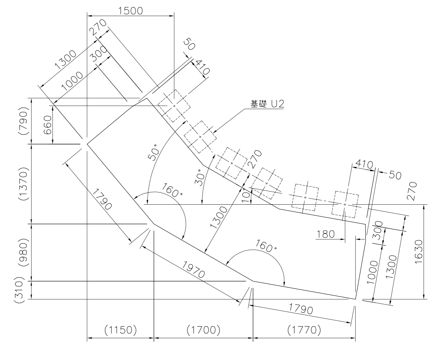
基礎伏図 S=1/40
