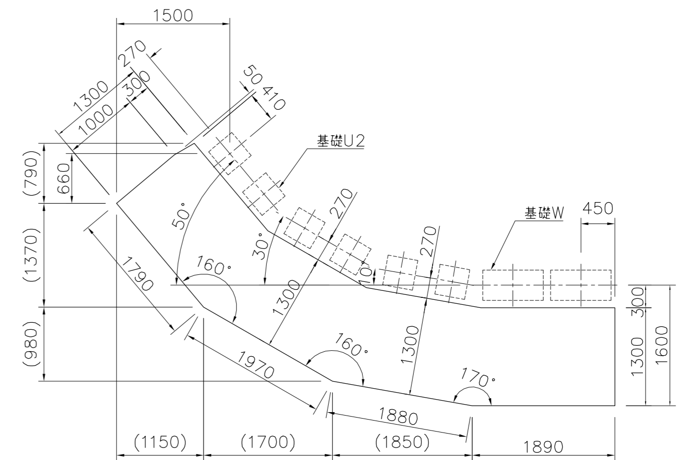
基礎伏図 S=1/50
