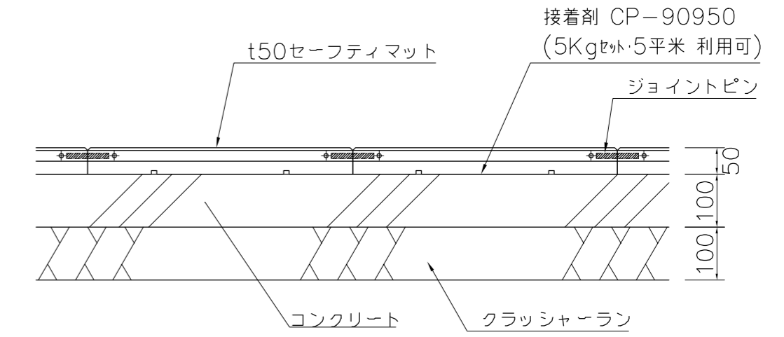
参考施工図 S=1/10
