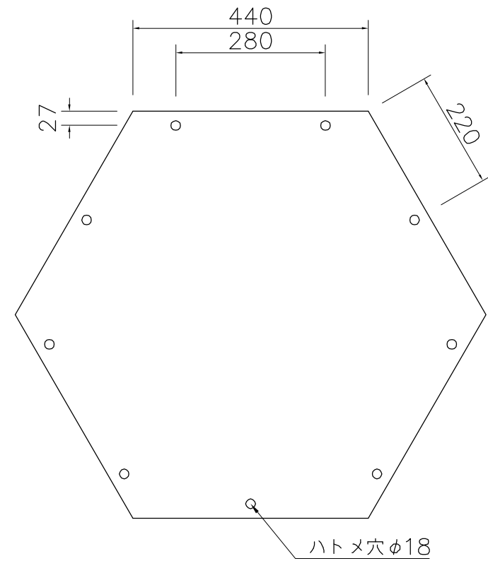
詳細図 S=1/10
